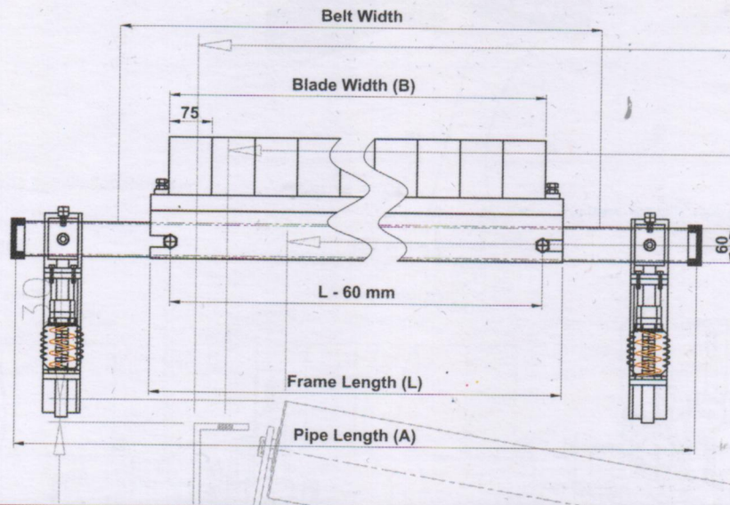
PU BLADE
